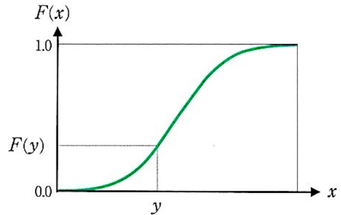
(a) 分布関数 F(x)
