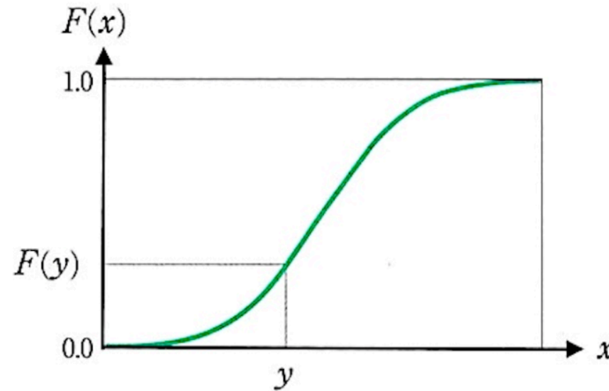
(a) 分布関数 F(x)
